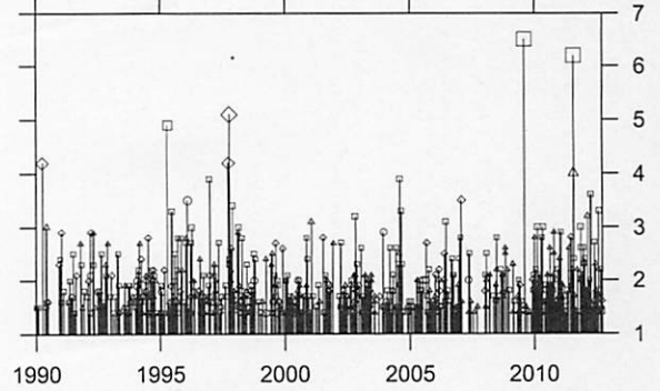
M-T 図
