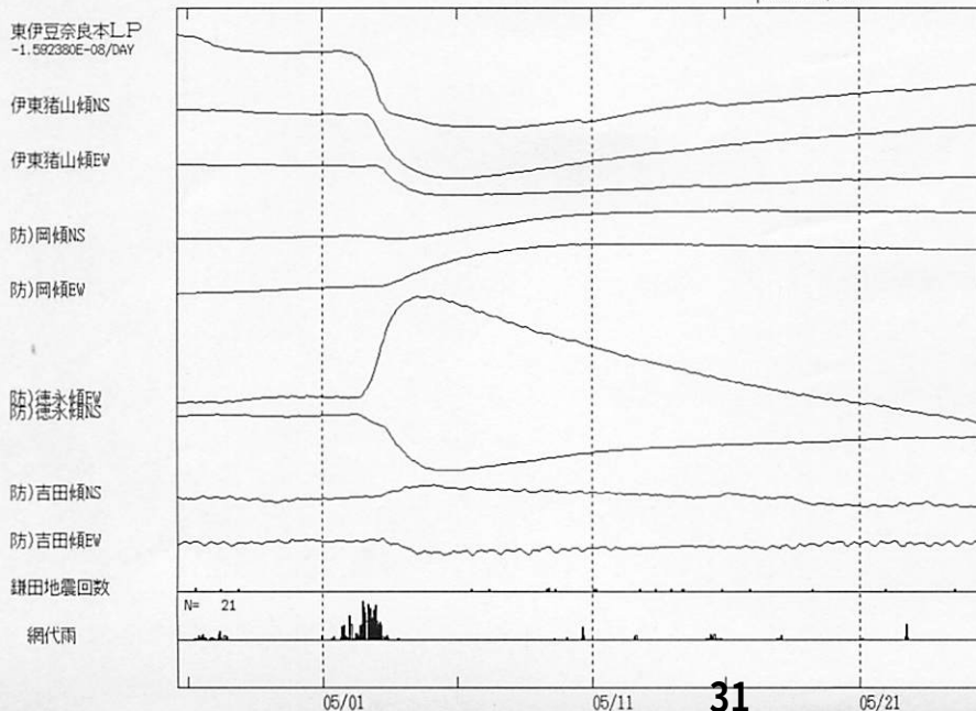
東伊豆地域の体積ひずみ計・傾斜計の記録 （2012年4月25日14時～5月25日14時）
