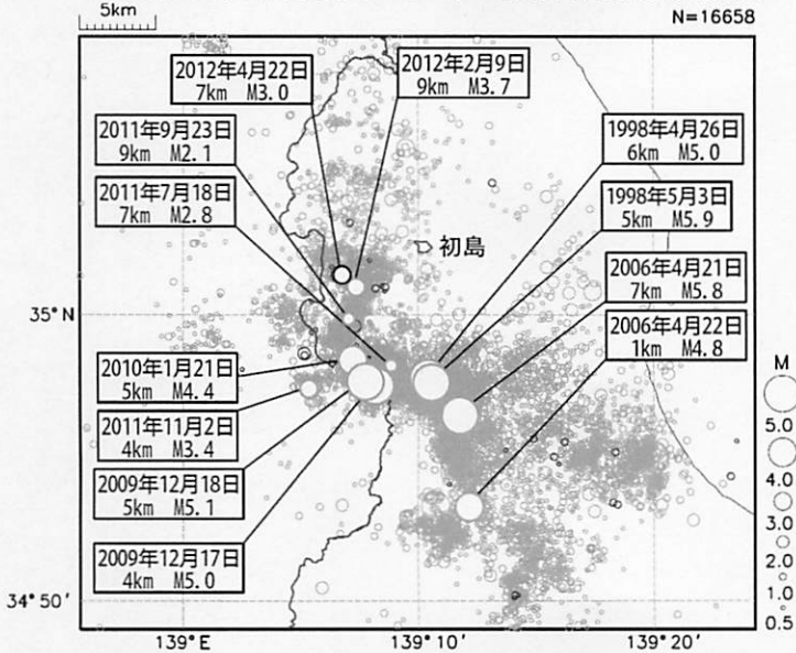
震央分布図（1997年10月1日～2012年5月23日、 M \geq 0.5 、深さ0～20km）
