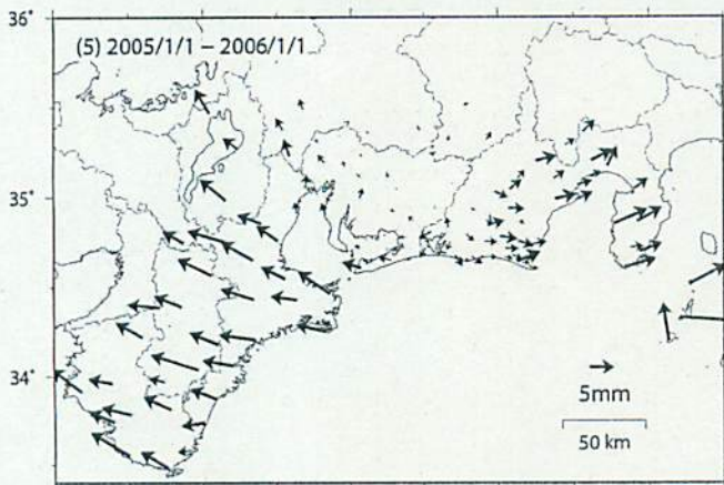
【水平変動】
