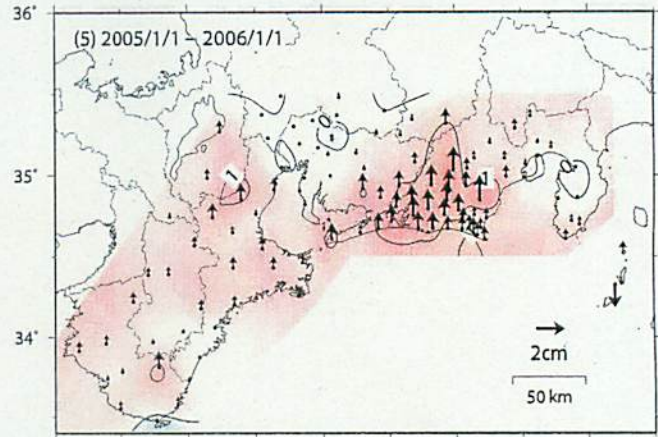
【上下変動】
