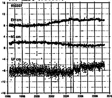
(5) 引佐 (93050)
