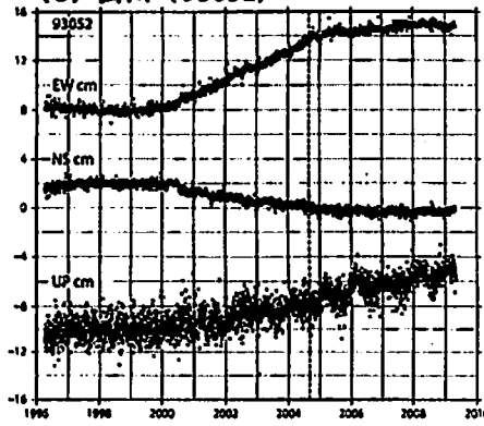
(8) 掛川 (93052)
