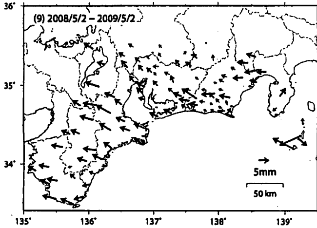
【水平変動】
