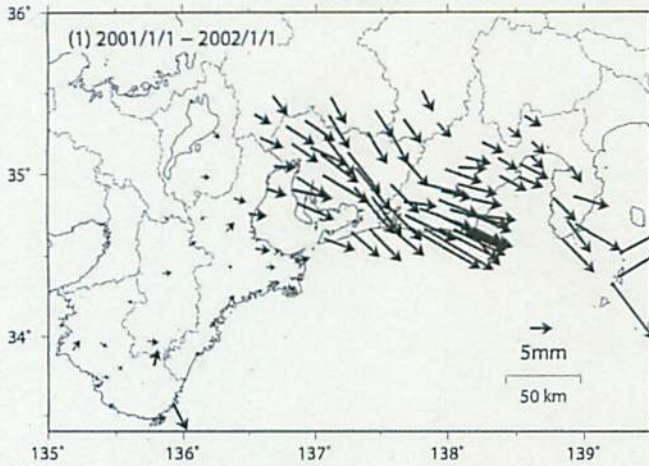
【水平変動】
