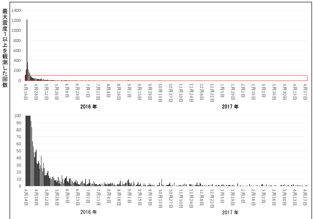
図1 震度1以上を観測した地震の日別回数グラフ（2016年4月14日～2017年4月30日） 下段は、上段の赤枠内（0回～100回の範囲）を拡大表示したもの
