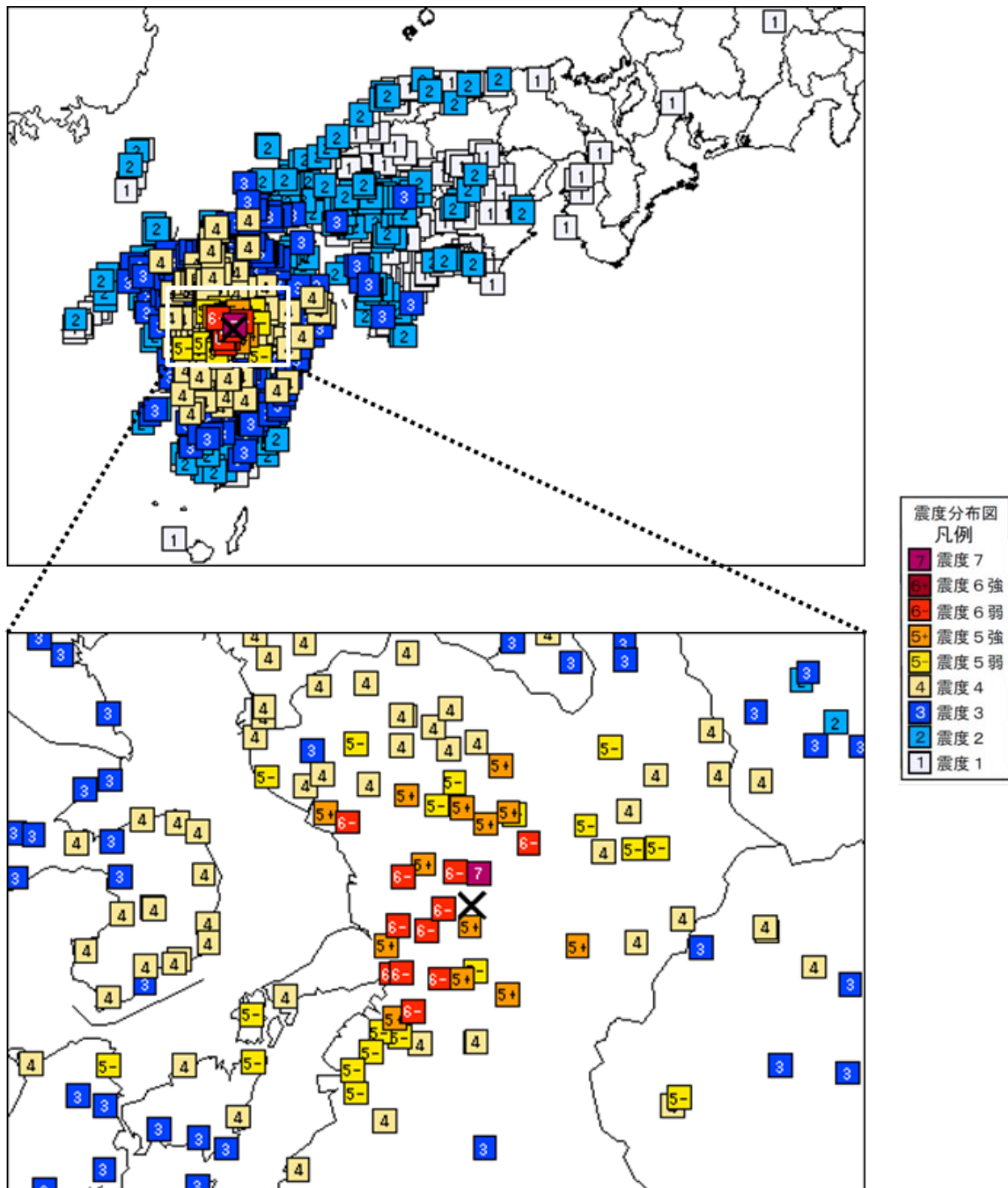
4月14日21時26分 熊本県熊本地方の地震（M6.5、深さ11km、最大震度7）の震度分布図 （×印は震央を示す。）
