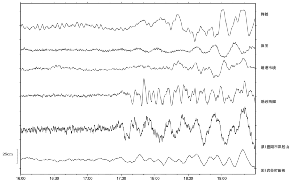
津波波形図
