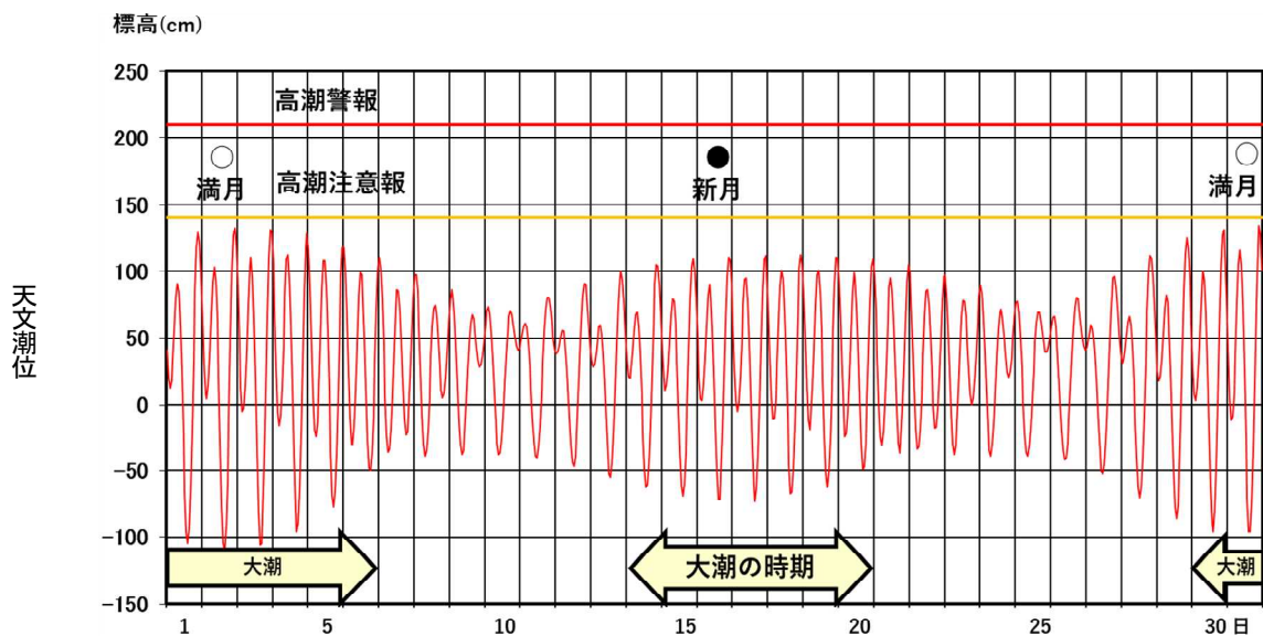
図3 大分における2023年8月（1時間ごとの）の天文潮位
