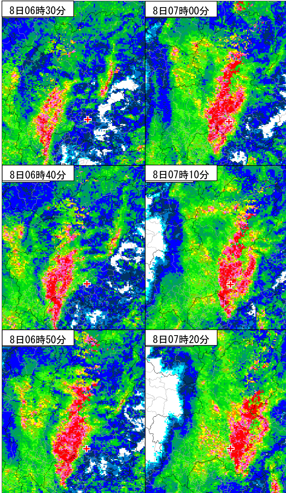
レーダーエコー強度 (mm/h) 0 1 2 4 8 12 16 24 32 40 48 56 64 80 レーダーエコー強度図 (合成レーダー) 令和2年7月8日06時30分～07時20分 図中 + 印は被害発生地域を示す。
