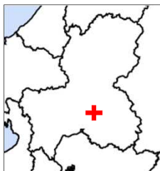
レーダーエコー強度 (mm/h) 0 1 2 4 8 12 16 24 32 40 48 56 64 80 レーダーエコー強度図 (合成レーダー) 令和2年7月8日06時30分～07時20分 図中 + 印は被害発生地域を示す。
