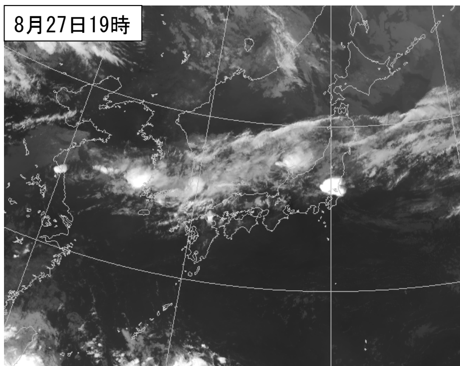
地上天気図及び気象衛星「ひまわり8号」が観測した赤外画像
