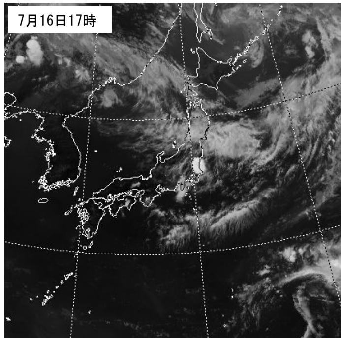
地上天気図及び気象衛星「ひまわり8号」赤外画像
