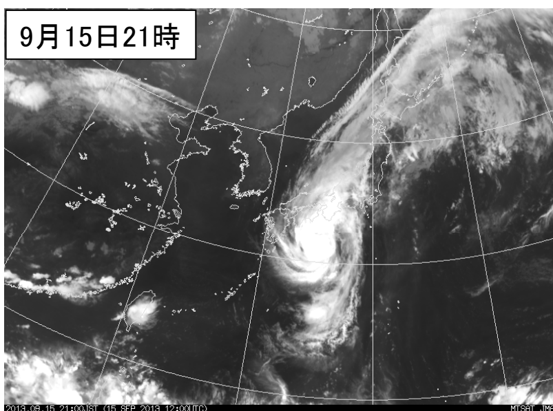
地上天気図および気象衛星「ひまわり7号」赤外画像
