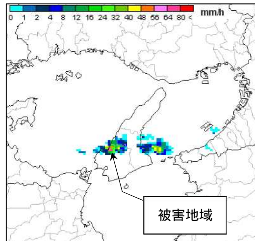
気象レーダー画像 (9月4日06時30分)
