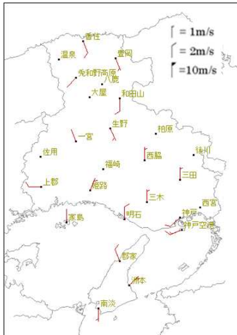
アメダス地点における風向風速分布図 (9月4日06時30分)
