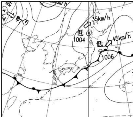
地上天気図 (9月4日06時)
