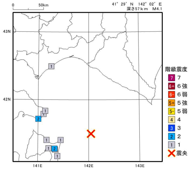
2024年3月14日18時37分 青森県東方沖の地震の震度分布図
