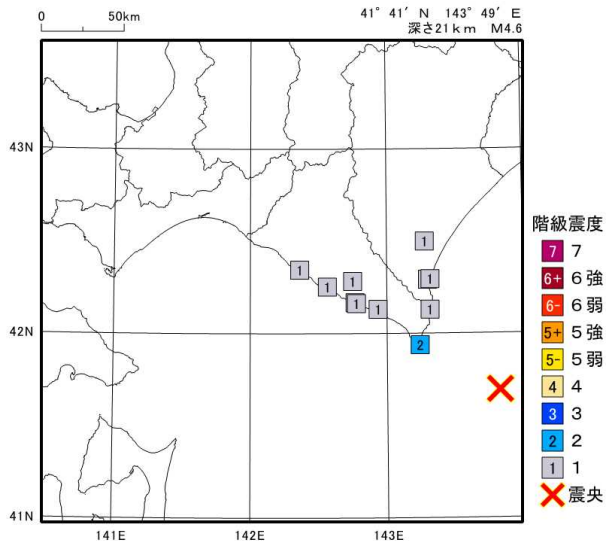
2024年3月19日10時15分 十勝沖の地震の震度分布図
