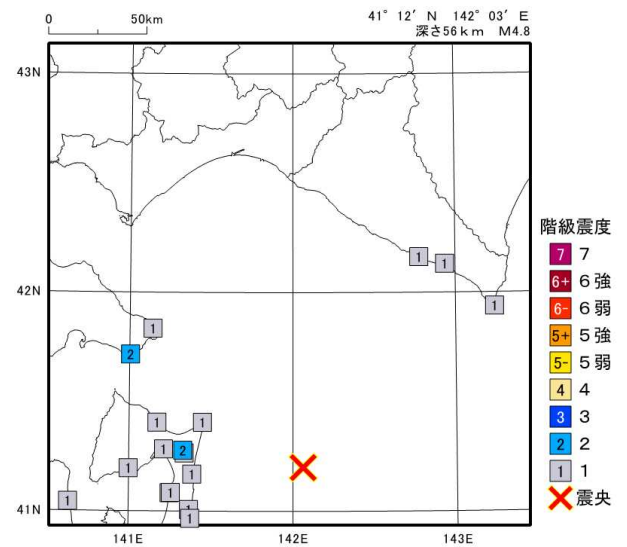
2024年 3月 3日17時31分 青森県東方沖の地震の震度分布図
