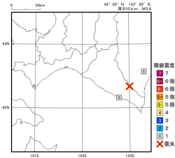
2024年 3月 1日16時04分 日高地方東部の地震の震度分布図
