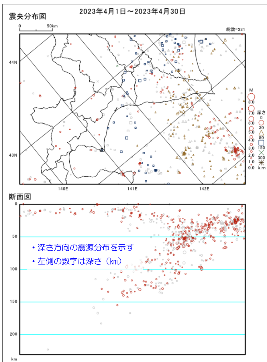
図2 断面図の例
