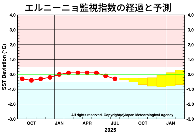
図 1 エルニーニョ監視海域の監視指数（海面水温の基準値との差）の 5 か月移動平均値の経過と予測 エルニーニョ監視海域の監視指数（海面水温の基準値との差）の 5 か月移動平均値について、7 月までの経過（観測値）を折れ線グラフで、大気海洋結合モデルによる予測結果（70%の確率で入ると予想される範囲）をボックスで示している。監視指数の 5 か月移動平均値が赤（+0.5℃以上）／青（-0.5℃以下）の範囲に入っている状態で 6 か月以上持続した場合に、エルニーニョ／ラニーニャ現象の発生としている。エルニーニョ監視海域の海面水温の基準値はその年の前年までの 30 年間の各月の平均値。
