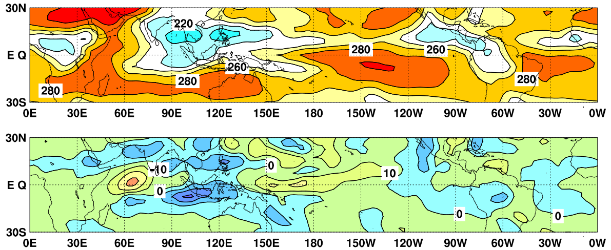
図 9 外向き長波放射量 (OLR) (上) 及び年間偏差 (下) の分布図 (2025 年 9 月)
