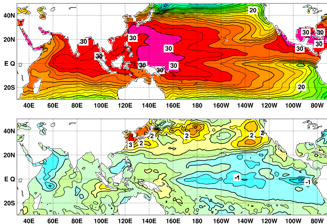
図4 2025年9月の海面水温図（上）及び平年偏差図（下）
