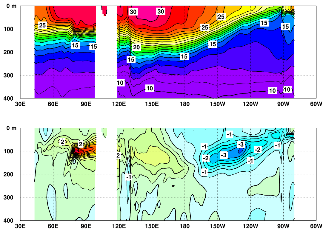
図5 2025年9月のインド洋から太平洋の赤道に沿った水温（上）及び平年偏差（下）の断面図
