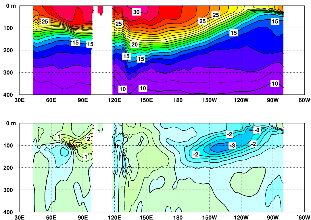
図5 2017年10月のインド洋から太平洋の赤道に沿った水温（上）及び平年偏差（下）の断面図
