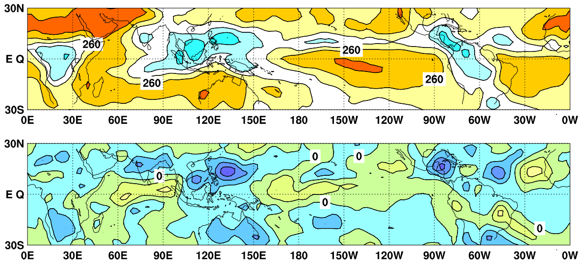
図 8 外向き長波放射量 (OLR) (上) 及び年平均偏差 (下) の分布図 (2017 年 10 月)
