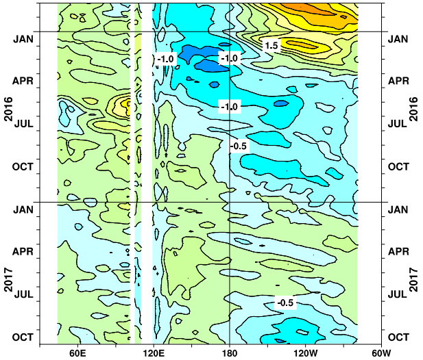
図 7 インド洋から太平洋の赤道に沿った海面から深度 300m までの平均水温年平均偏差の経度-時間断面図
