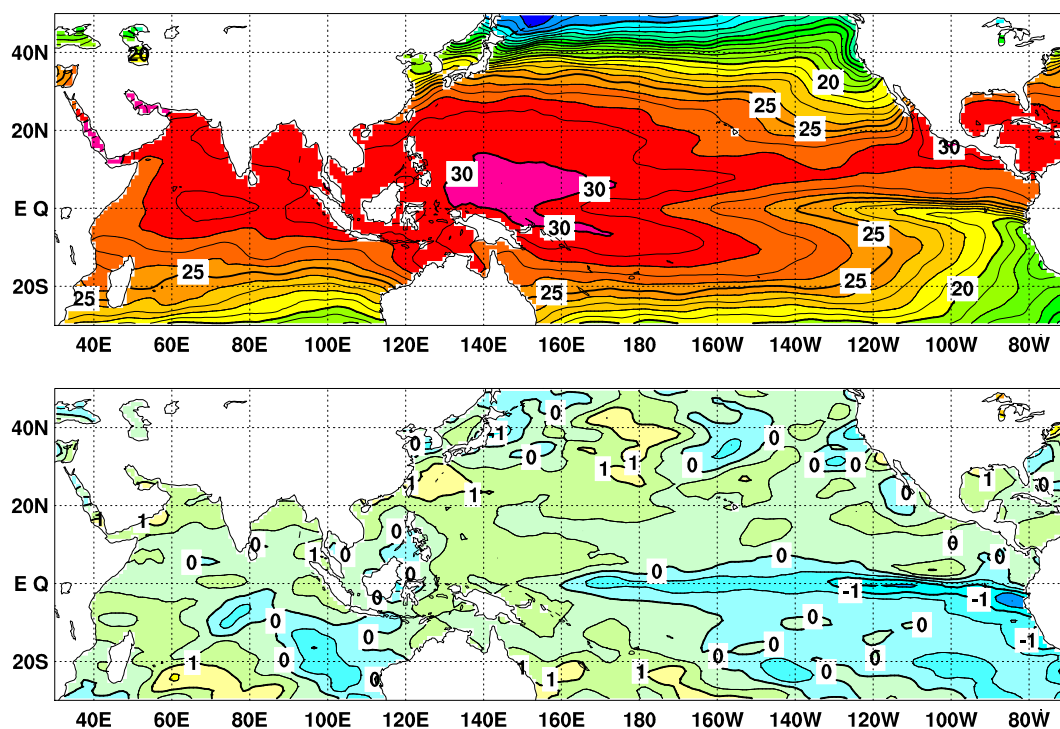
図4 2017年10月の海面水温図（上）及び平年偏差図（下）
