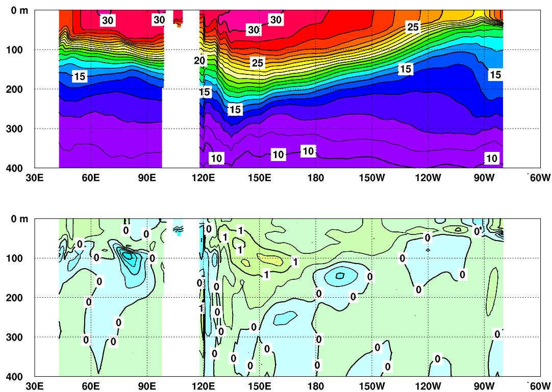
図5 2017年6月のインド洋から太平洋の赤道に沿った水温（上）及び平年偏差（下）の断面図
