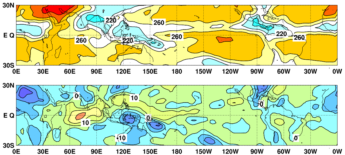
図 8 外向き長波放射量 (OLR) (上) 及び年偏差 (下) の分布図 (2017 年 6 月)
