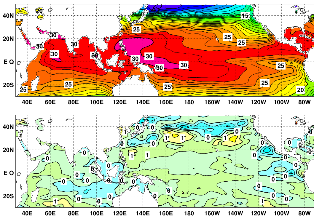
図4 2017年6月の海面水温図（上）及び平年偏差図（下）
