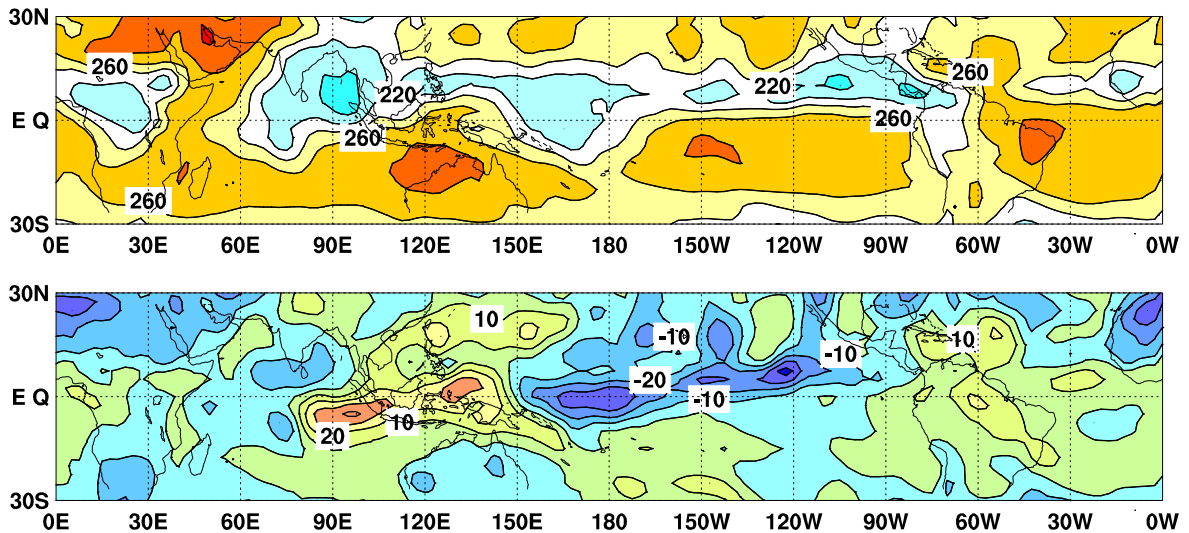
図6 外向き長波放射量 (OLR) (上) 及び年偏差 (下) の分布図 (2015年9月)
