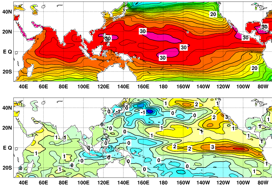
図 2 2015 年 9 月の海面水温図 (上) 及び平年偏差図 (下)
