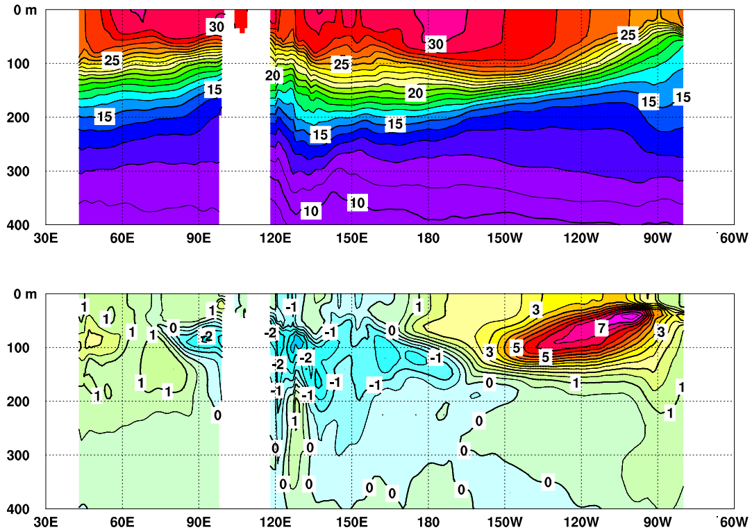
図 3 2015 年 9 月のインド洋から太平洋の赤道に沿った水温 (上) 及び平年偏差 (下) の断面図
