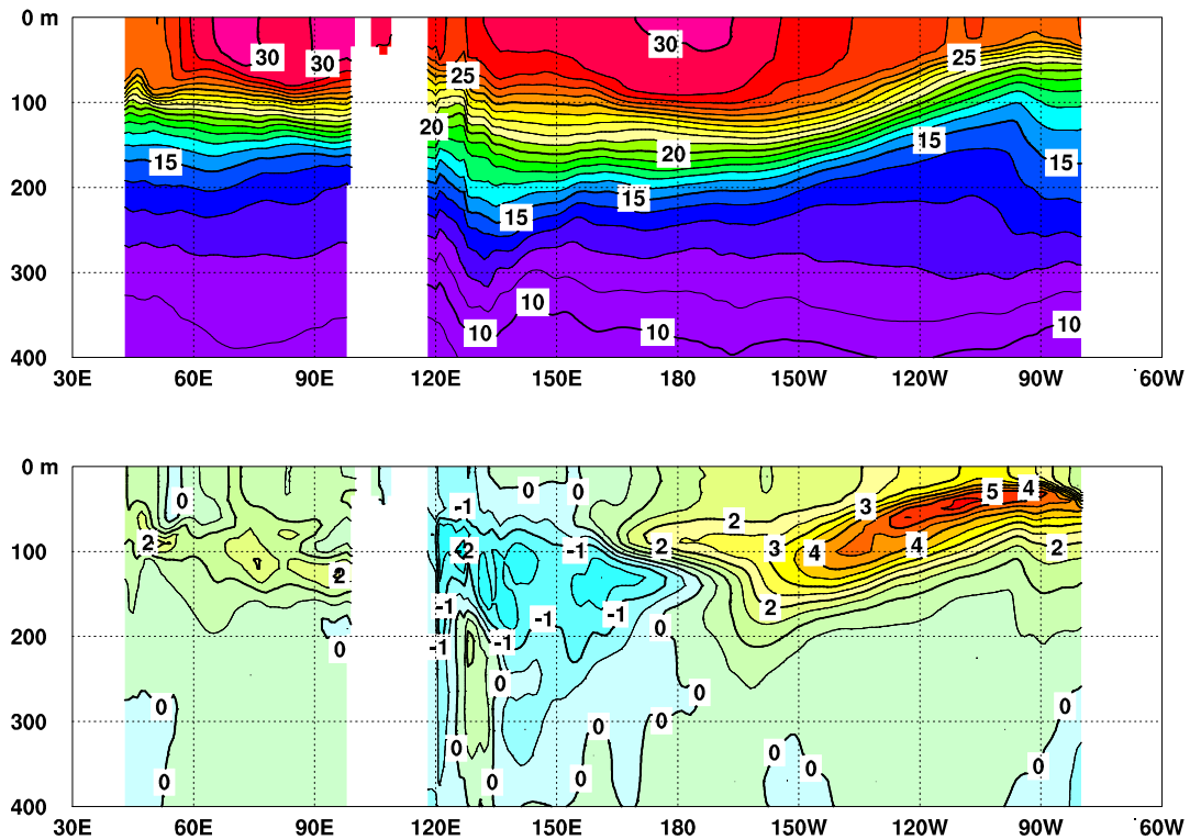
図 3 2015 年 7 月のインド洋から太平洋の赤道に沿った水温 (上) 及び平年偏差 (下) の断面図
