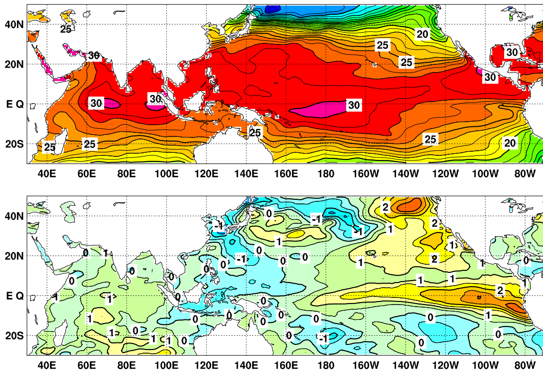
図 2 2015 年 7 月の海面水温図 (上) 及び平年偏差図 (下)
