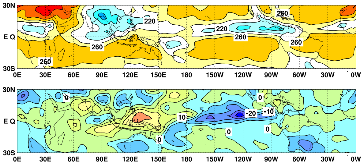
図6 外向き長波放射量 (OLR) (上) 及び年偏差 (下) の分布図 (2015年7月)
