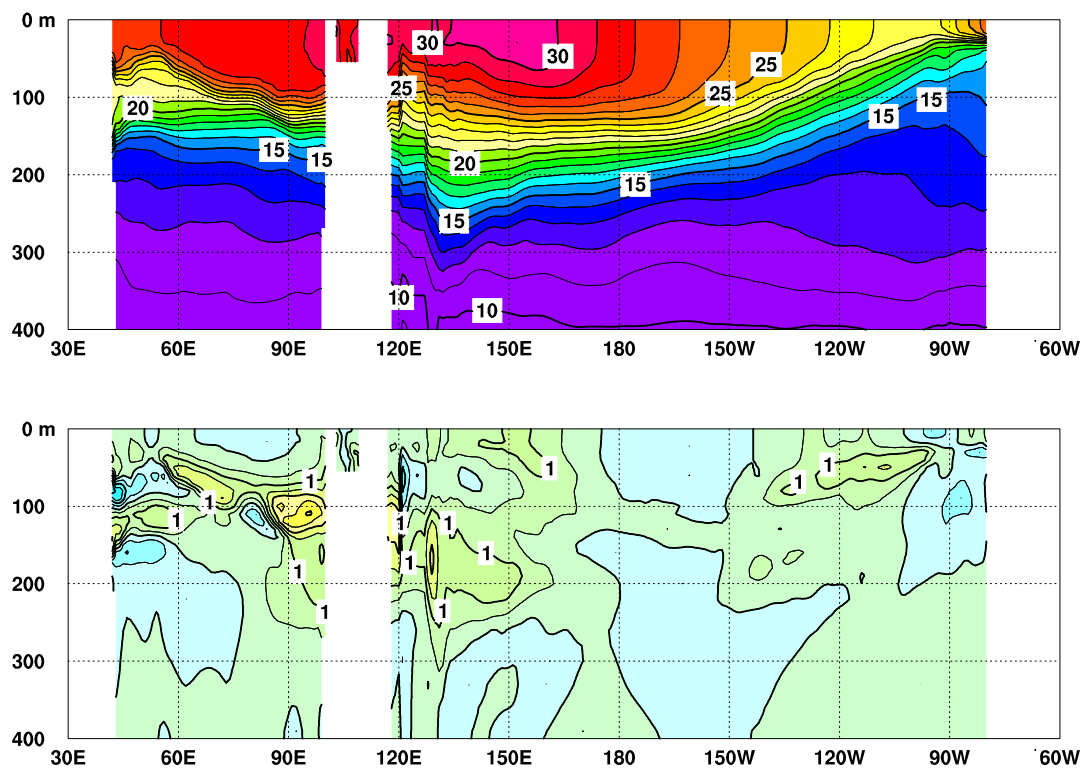
図 3 2013 年 12 月のインド洋から太平洋の赤道に沿った水温 ( 上 ) 及び平年偏差 ( 下 ) の断面図
