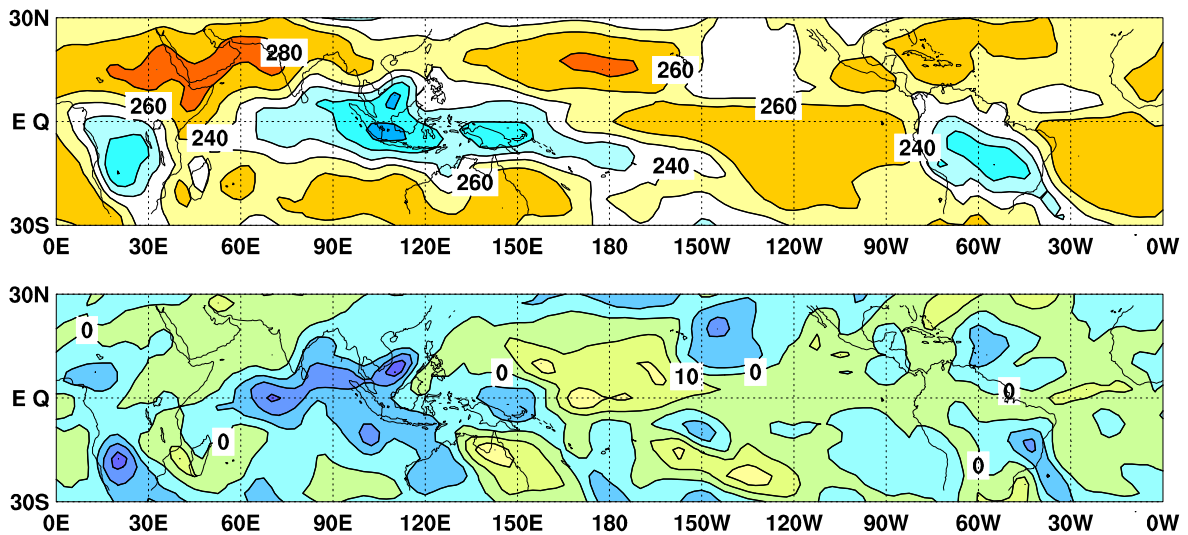
図6 外向き長波放射量(OLR)(上)及び年偏差(下)の分布図(2013年12月)
