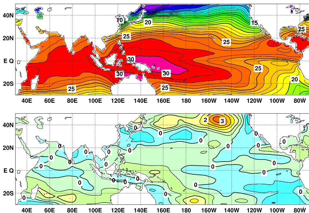
図 2 2013 年 12 月の海面水温図 ( 上 ) 及び平年偏差図 ( 下 )
