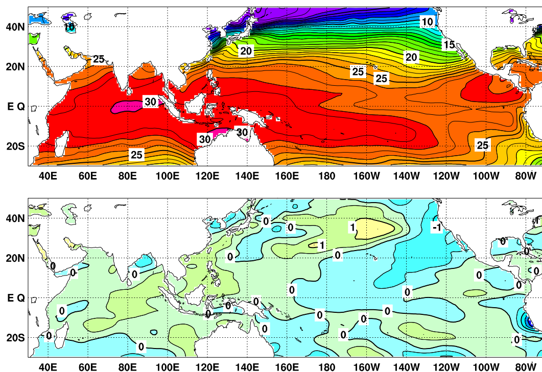
図 2 2013 年 3 月の海面水温図 ( 上 ) 及び平年偏差図 ( 下 )
