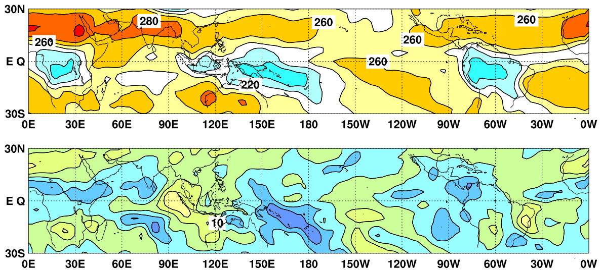
図6 外向き長波放射量 (OLR) (上) 及び年偏差 (下) の分布図 (2013 年 3 月)
