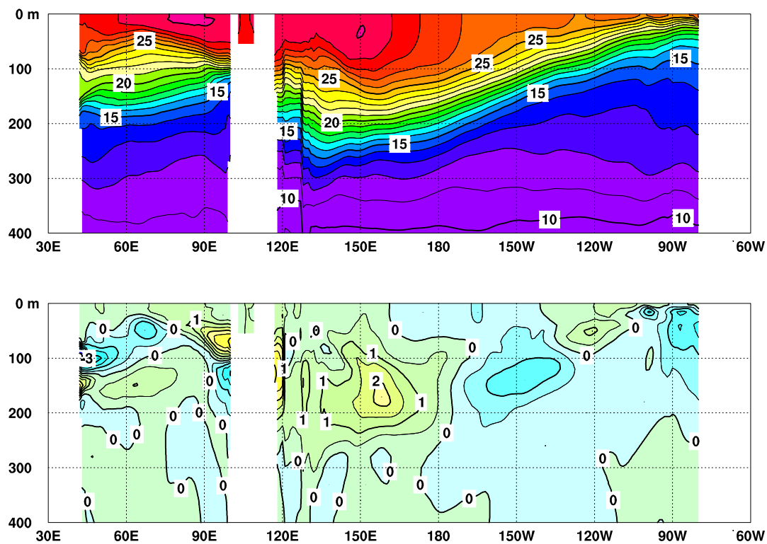
図 3 2013 年 3 月のインド洋から太平洋の赤道に沿った水温 ( 上 ) 及び平年偏差 ( 下 ) の断面図
