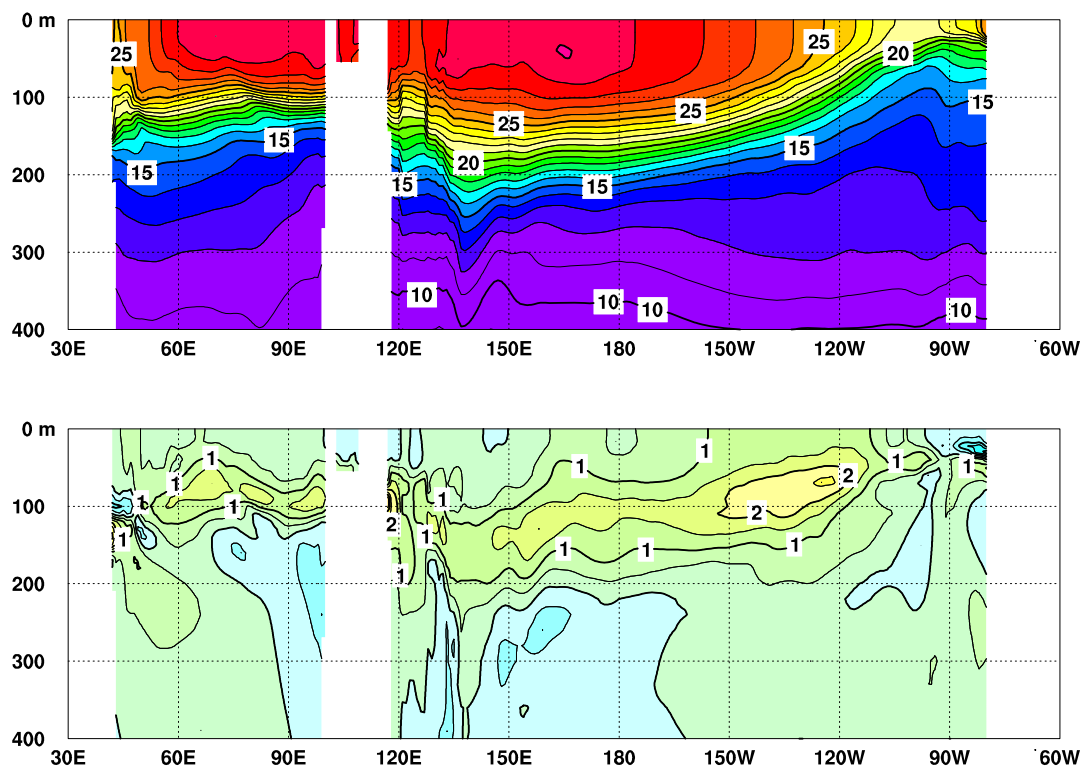
図 3 2012 年 8 月のインド洋から太平洋の赤道に沿った水温 ( 上 ) 及び平年偏差 ( 下 ) の断面図
