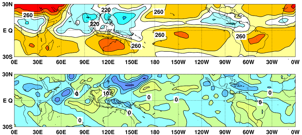
図6 外向き長波放射量 (OLR) (上) 及び年偏差 (下) の分布図 (2012 年 8 月)
