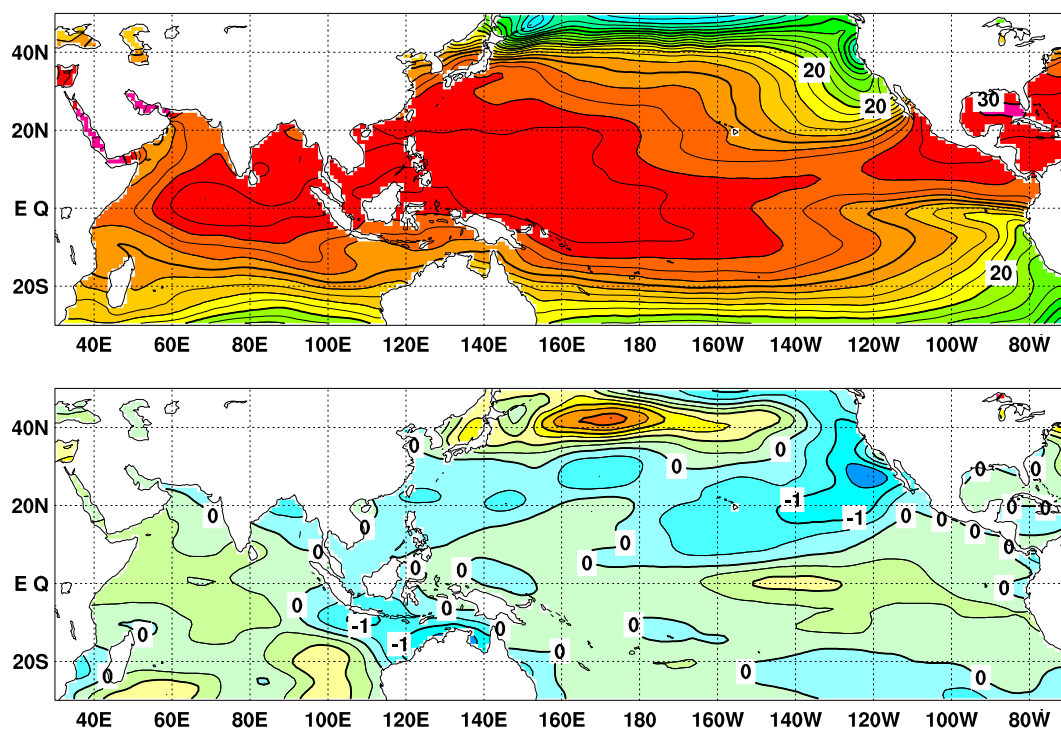
図 2 2012 年 8 月の海面水温図 ( 上 ) 及び平年偏差図 ( 下 )
