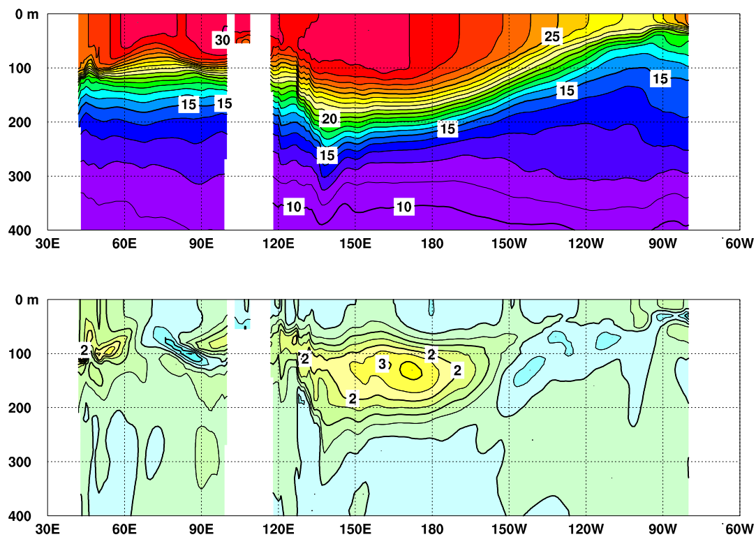
図 3 2011 年 7 月のインド洋から太平洋の赤道に沿った水温 ( 上 ) 及び平年偏差 ( 下 ) の断面図
