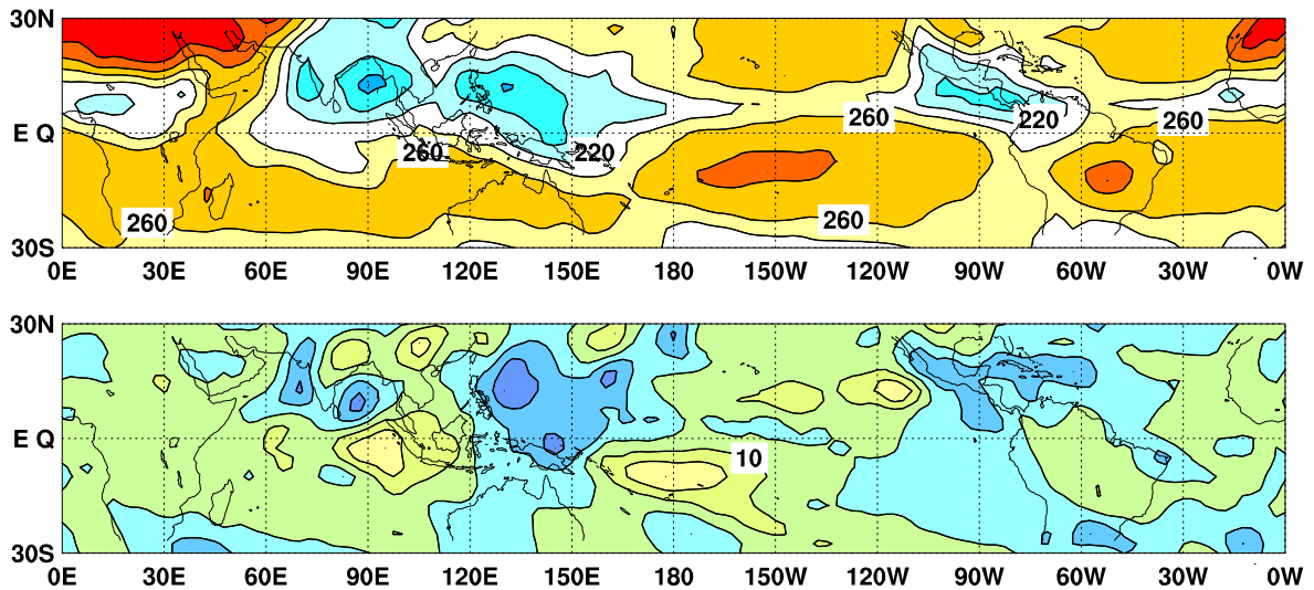
図6 外向き長波放射量 (OLR) (上) 及び年偏差 (下) の分布図 (2011 年 7 月)
