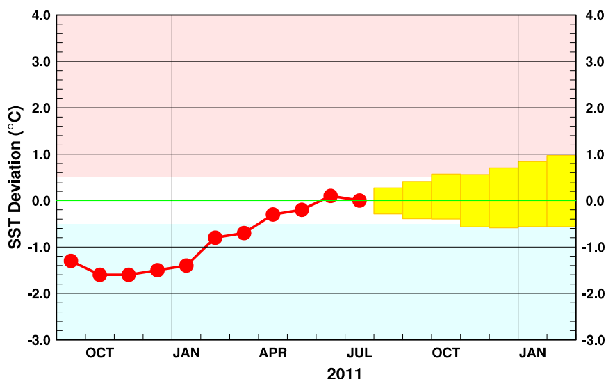
図9 エルニーニョ監視海域の海面水温の基準値との差の先月までの経過 (折れ線グラフ) とエルニーニョ予測モデルから得られた今後の予測 (ボックス)
