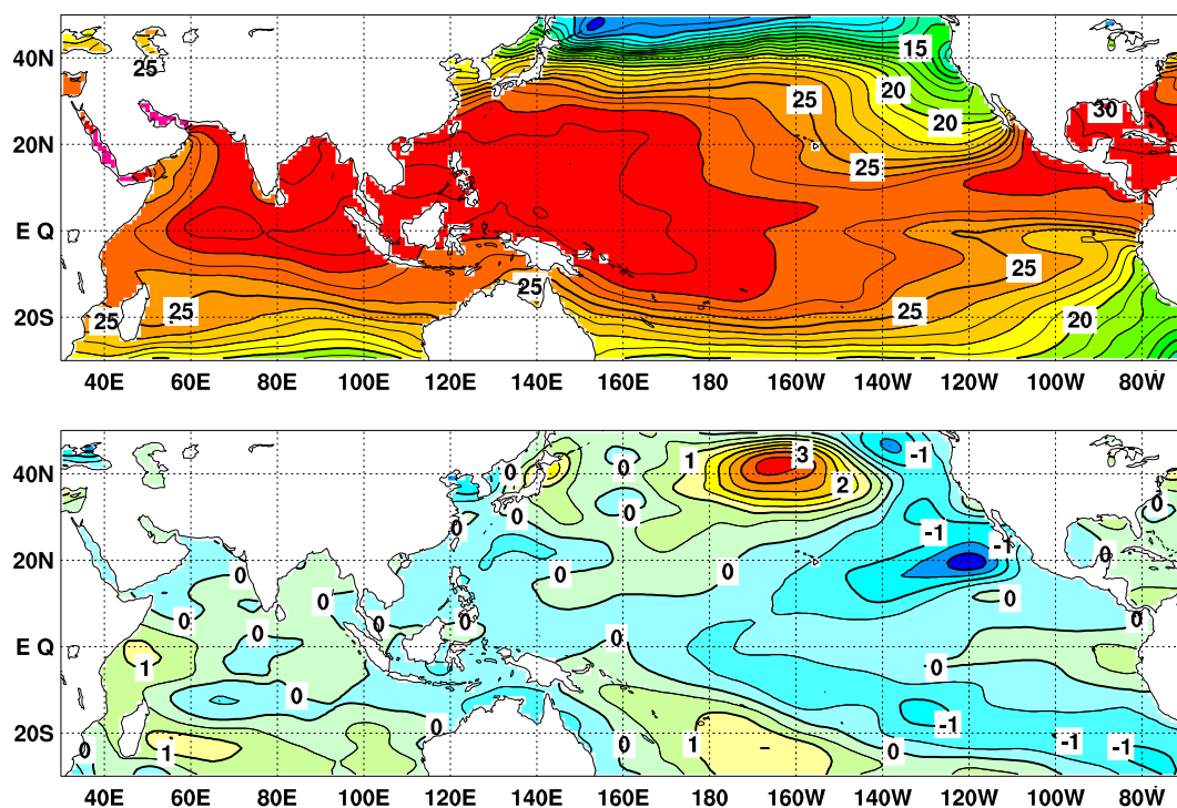
図 2 2011 年 7 月の海面水温図 ( 上 ) 及び平年偏差図 ( 下 )
