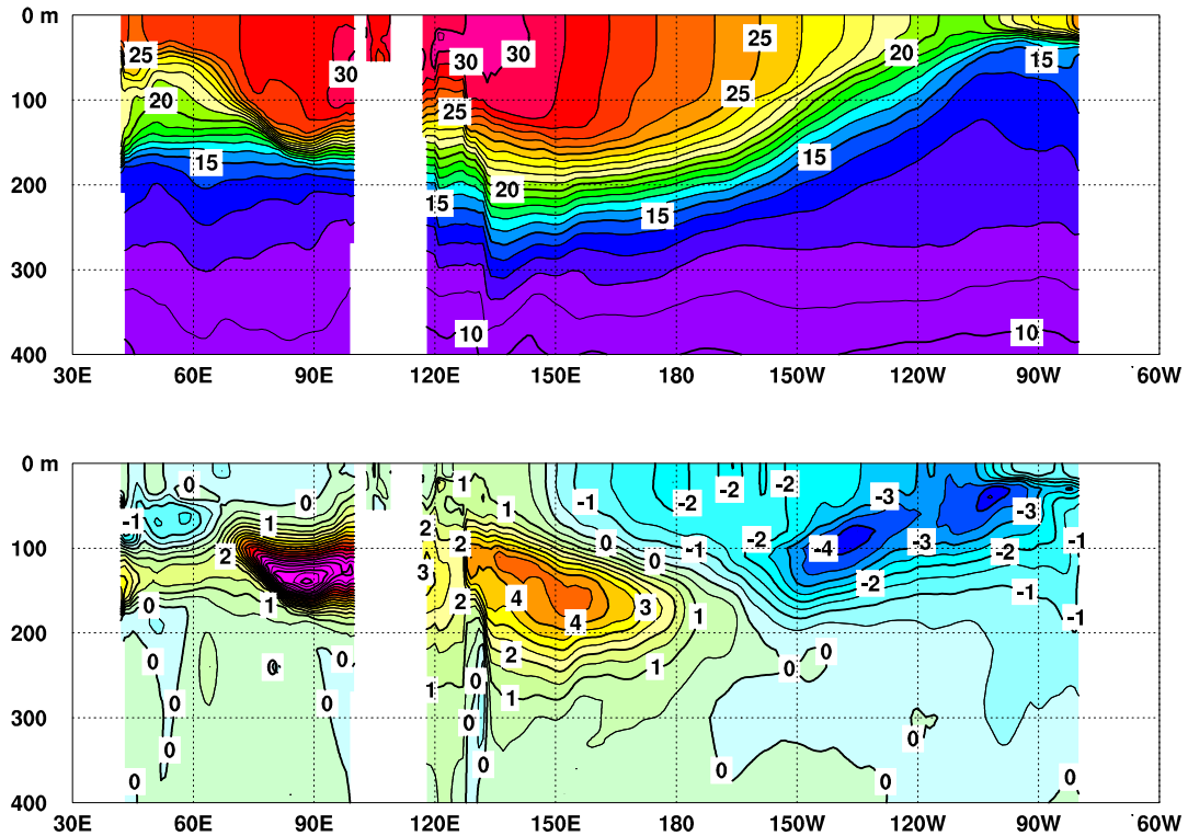
図 3 2010 年 12 月のインド洋から太平洋の赤道に沿った水温 ( 上 ) 及び年偏差 ( 下 ) の断面図
