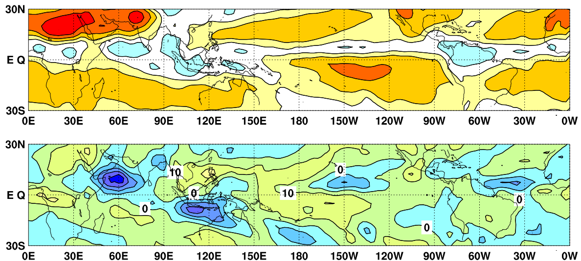
図6 外向き長波放射量 (OLR) (上) 及び年偏差 (下) の分布図 (2010 年 5 月)
