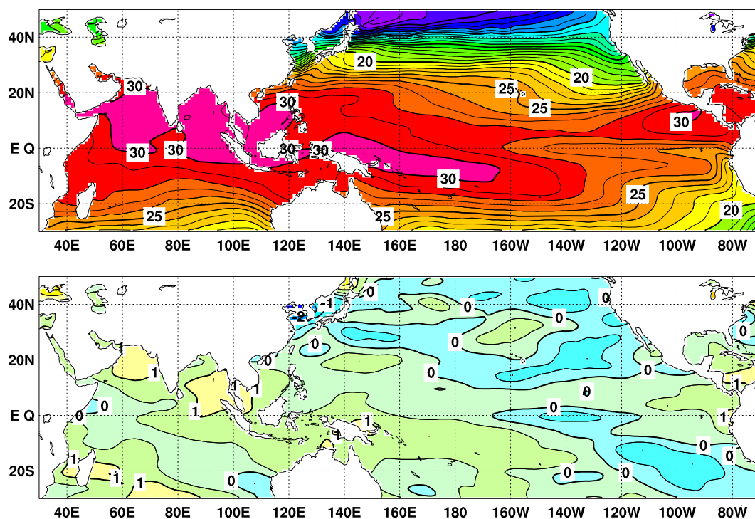
図 2 2010 年 5 月の海面水温図 ( 上 ) 及び 年 平 年 偏 差 図 ( 下 )
