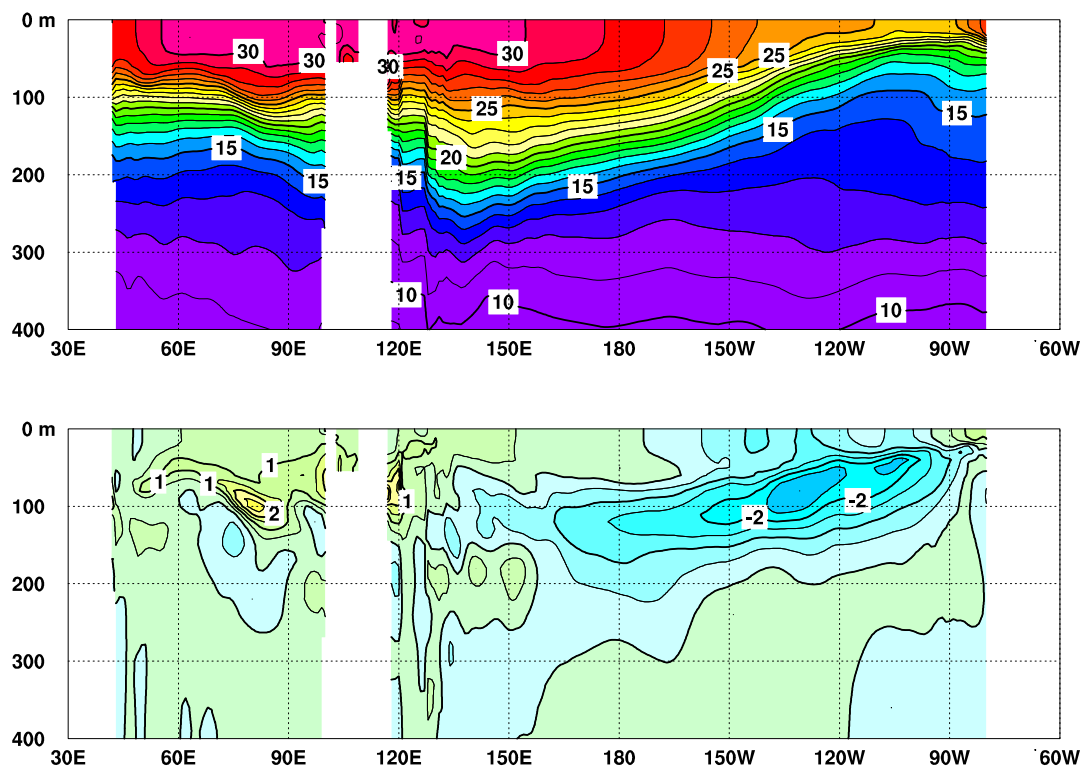
図 3 2010 年 5 月のインド洋から太平洋の赤道に沿った水温 ( 上 ) 及び 年 平 年 偏 差 ( 下 ) の 断 面 図
