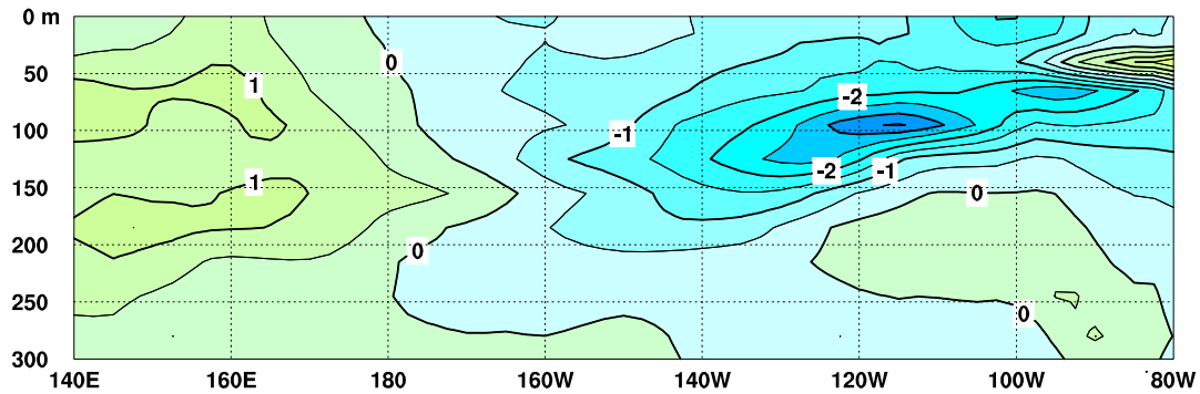
図 3 2005 年 11 月の太平洋の赤道に沿った水温 (上) 及び年平均偏差 (下) の断面図 (海洋データ同化システムによる)。上図の等値線間隔は 1^{\circ}\text{C} 、下図の等値線間隔は 0.5^{\circ}\text{C} (年平均値は 1987 ~ 2004 年の 18 年平均値)。
