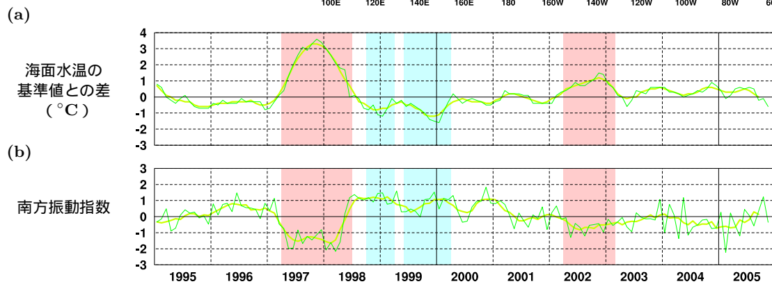
図1 エルニーニョ監視海域の海面水温の基準値との差 ( ^{\circ}\text{C} ) (a) と南方振動指数 (b) の推移 (1995年1月～2005年11月)。折線は月平均値、滑らかな太線は5か月移動平均値を示す (海面水温の基準値は1961～1990年の30年平均値、南方振動指数の年平均値は1971～2000年の30年平均値)。赤色の陰影はエルニーニョ現象の発生期間を、青色の陰影はラニーニャ現象の発生期間を示している。
