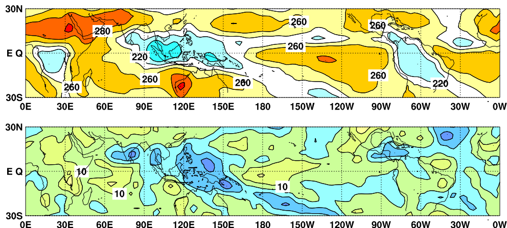
図6 2005年11月の外向き長波放射量(OLR)(上)及び平年偏差(下)の分布図。OLRの値が小さいほど、対流活動が活発であることを示す。上図は 20\text{W}/\text{m}^2 毎、下図は 10\text{W}/\text{m}^2 毎に等値線を描いている(平年値は1979～2000年の22年平均値)。OLRデータは米国海洋大気庁(NOAA)から提供されたものである。
