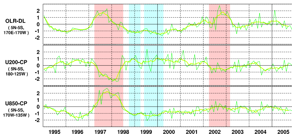
図7 日付変更線付近のOLR指数(OLR-OL)、対流圏上層(200hPa)の赤道東西風指数(U200-CP)、対流圏下層(850hPa)の赤道東西風指数(U850-CP)の時系列(上から順に)。折線は月平均値、滑らかな太線は5か月移動平均値を示す(平年値は1979～2000年の22年平均値)。赤色の陰影はエルニーニョ現象の発生期間を、青色の陰影はラニーニャ現象の発生期間を示している。
