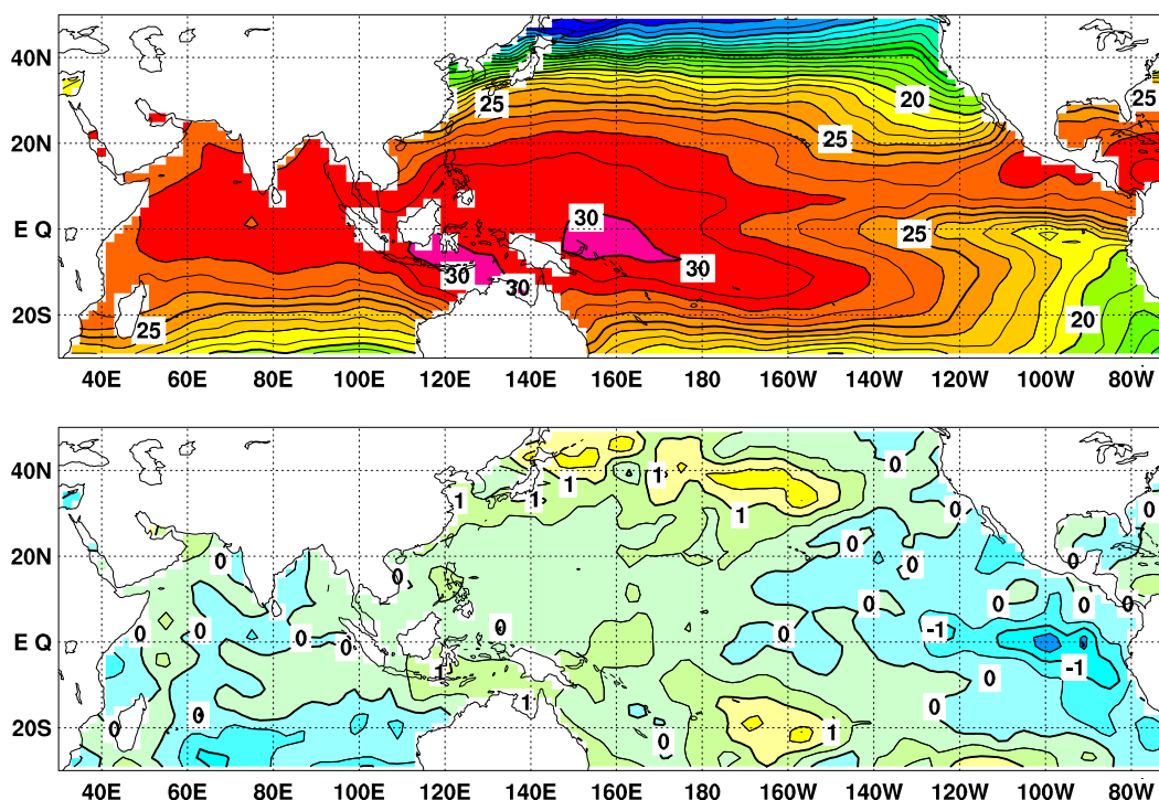
図2 2005年11月の海面水温図(上)及び平年偏差図(下)。海面水温図の太線は 5^{\circ}\text{C} 毎、細線は 1^{\circ}\text{C} 毎、平年偏差図の太線は 1^{\circ}\text{C} 毎、細線は 0.5^{\circ}\text{C} 毎の等値線を示す(平年値は1971~2000年の30年平均値)。
