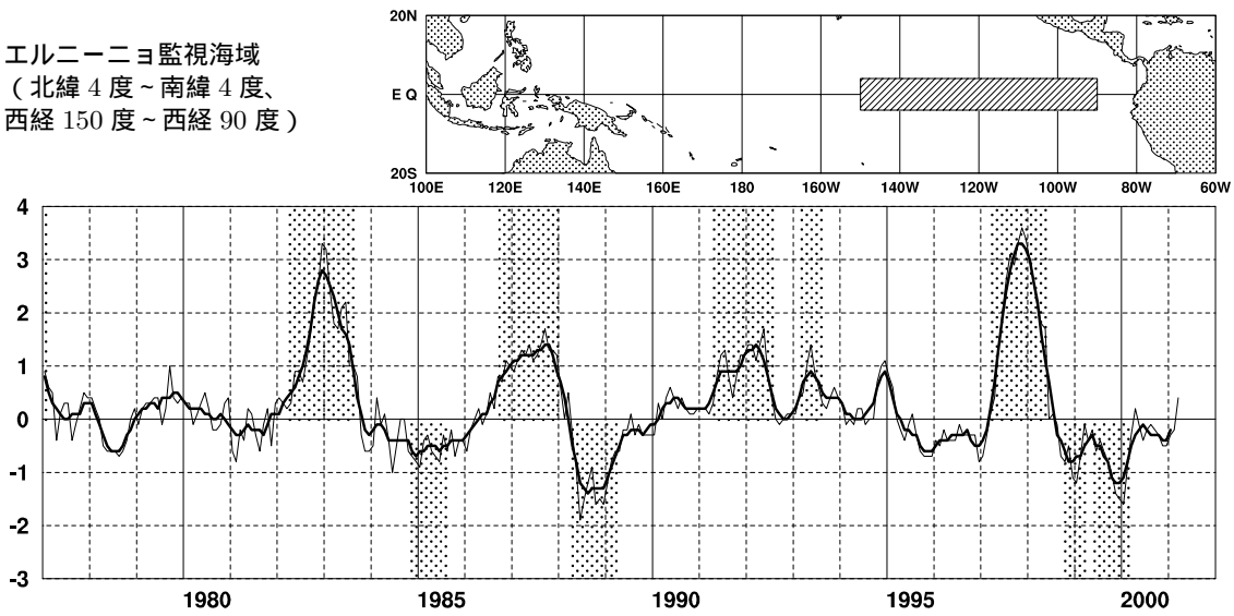
図 1 エルニーニョ監視海域の月平均海面水温の基準値との差 (°C) の推移 (1977 年 1 月 ~ 2001 年 3 月)。折線は月平均値、滑らかな太線は 5 か月移動平均値を示し、正の値は基準値より高いことを示す。エルニーニョ現象の発生期間は上側に、ラニーニャ現象の発生期間は下側に、それぞれ陰影を施してある (基準値は 1961 ~ 1990 年の 30 年平均値)。
