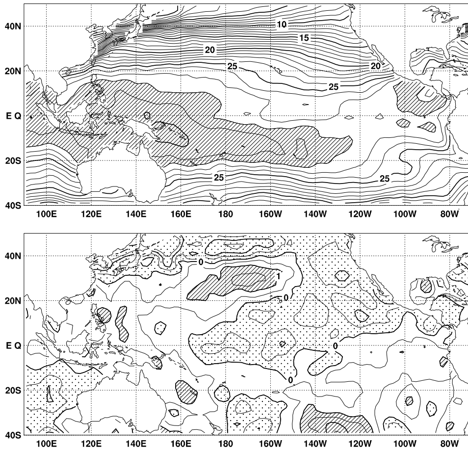
図 2 2001 年 3 月の海面水温図 (上) 及び平年偏差図 (下)。海面水温図の大線は 5°C 毎、細線は 1°C 毎の、平年偏差図の大線は 1°C 毎、細線は 0.5°C 毎の等値線を示す。海面水温図の陰影部は 28°C 以上の領域を、偏差図の濃い (薄い) 陰影部は +1°C 以上の正偏差域 (0°C 以下の負偏差域) を示す (平年値は 1971 ~ 2000 年の 30 年平均値)。
