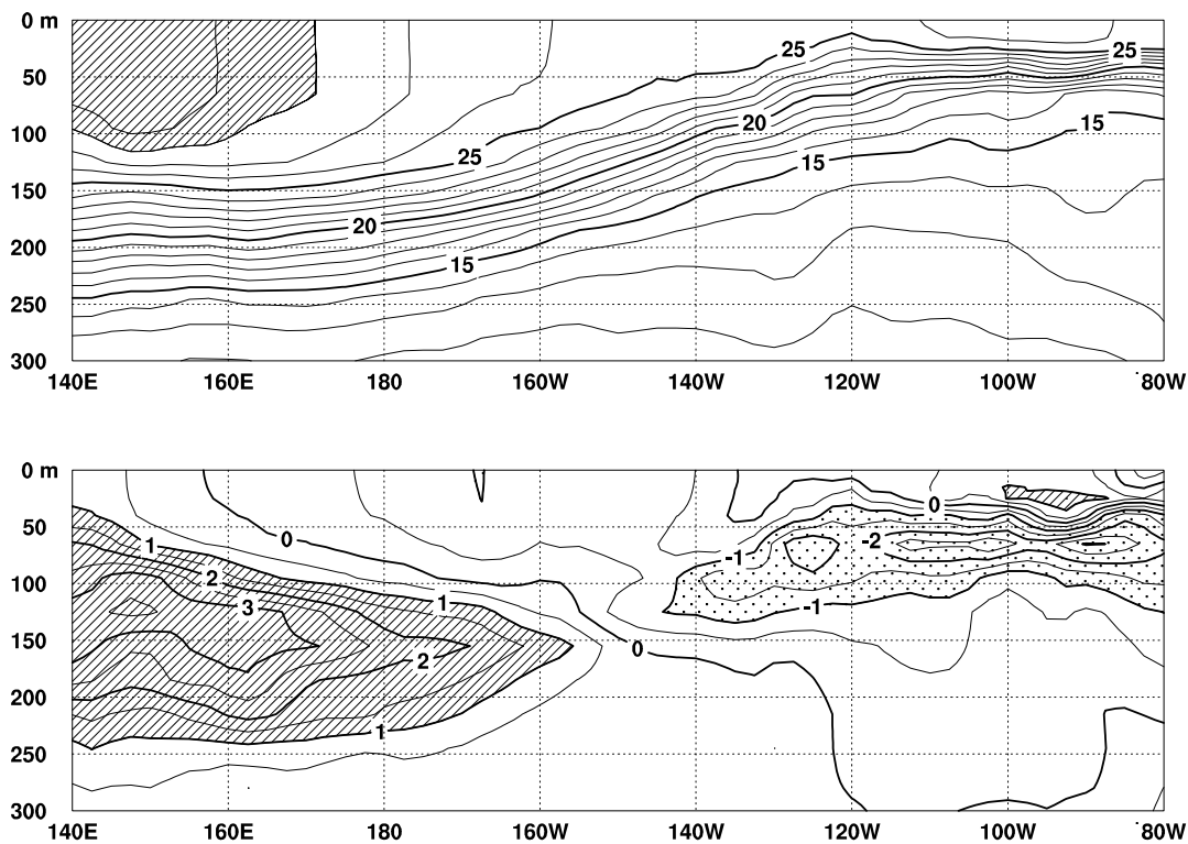
図3 2001年3月の太平洋の赤道に沿った水温(上)及び平年偏差(下)の断面図(海洋データ同化システムによる)。上図の等値線間隔は 1^{\circ}\text{C} で 28^{\circ}\text{C} 以上には陰影を施し、下図の等値線間隔は 0.5^{\circ}\text{C} で +1^{\circ}\text{C} 以上( -1^{\circ}\text{C} 以下)の偏差には濃い(薄い)陰影を施した(平年値は1987~1999年の13年平均値)。
