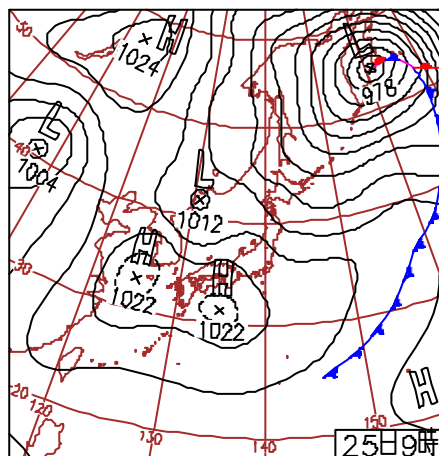
25日(日)全国的に晴れて気温低め 北日本の一部は寒気による雪や雨が残るが、その他は日本の南の高気圧に覆われて、ほぼ全国的に晴れ。北・東日本の最高気温は、平年より3～8度低く、4月上旬並。
