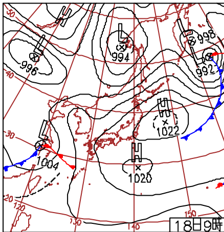
18日(日)青森で桜が開花 気圧の谷の影響で九州は雨。その他は晴れ。日本海側を中心に気温が上昇し、兵庫県豊岡市の最高気温は31.6。青森で桜開花。今期の桜開花は3/17に始まり約一ヶ月で青森へ。
