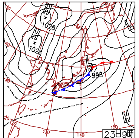
23日(金)日本海側で寒暖差大 寒冷前線が通過し寒気が入り、日本海側や南西諸島は雨。東北南部～東日本、山陰の最高気温は前日より約10度低く、新潟県高田市では13.9 低い15.5。
