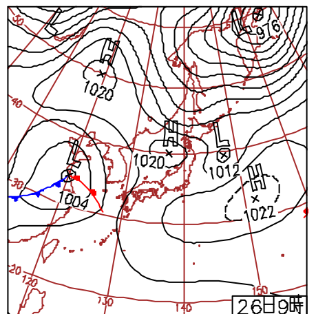
26日(月)西日本で大雨 上海付近の低気圧が発達しながら東北東進。日中はほぼ全国的に晴れるが、西日本は午後から雨。長崎県厳原町では48.5mm/hの激しい雨を伴い日雨量165mm。函館で桜が開花。
