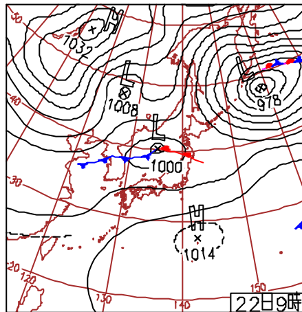
22日(木)各地で最高気温極値更新 低気圧が日本海を東進。東北部や北海道は曇りや雨、その他は晴れ。南から暖かい空気が入り、東・西日本を中心に気温が上がる。東京など各地で4月の最高気温を更新。
