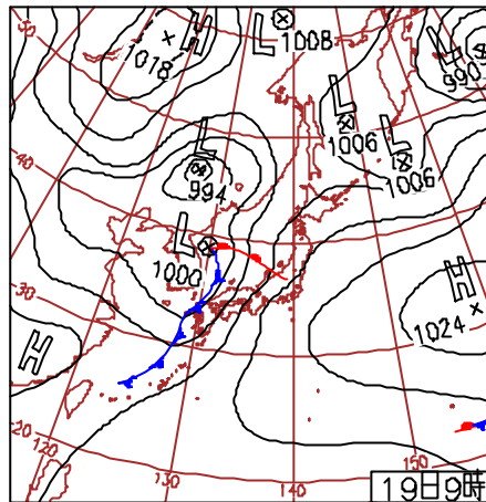
19日(月)寒冷前線通過で大荒れ 低気圧が発達しながら日本海を北東進し、寒冷前線が日本列島を東進。前線の通過に伴い室戸岬では最大風速23.4m/sの暴風。石垣島の伊原間では90mm/hの猛烈な雨。
