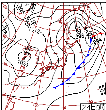
24日(土)北日本「寒の戻り」 冬型の気圧配置。北日本の上空約5500mには-33以下の寒気が入り、北海道の日本海側や東北～北陸の山沿いで雪。朝9時までの降雪量は青森県酸ヶ湯で19cm。
