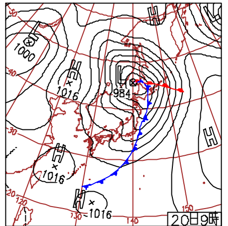
20日(火)仙台で瞬間風速33.3m/s 日本海の低気圧が発達しながらオホーツク海に進み、北日本は雨で風が強い。東日本～南西諸島は日中晴れて気温上昇。静岡の最高気温は4月の極値を更新する31.0。
