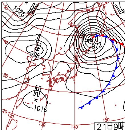
21日(水)羅臼で強風被害 発達した低気圧がオホーツク海をゆっくりと東北東進し、北日本の強風は次第に弱まる。北海道羅臼町では局地的な強風被害。北海道の一部で雨や雪の他は、全国的に概ね快晴。
