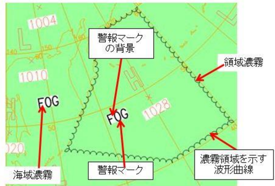
図6. 海上悪天予想情報の例 (その1) FSAS24/48 での描画
