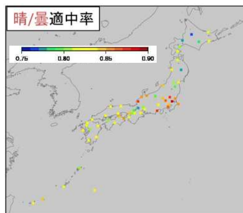
図8: 晴/曇 適中率
